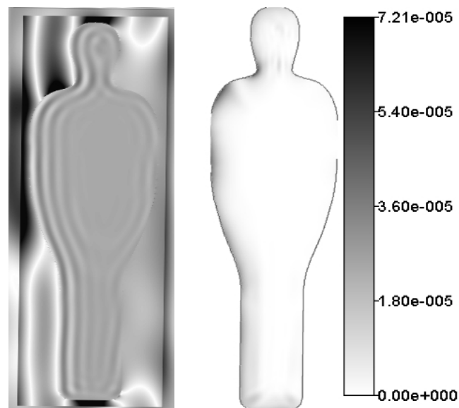
Рис. 2.8 Распределение поля (слева) и SAR (справа), однородная модель человека облучается плоской волной Е-поляризации на частоте 900МГц
