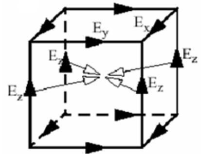
Рис. 3.4 Поясняющий рисунок к вычислению 12-ти точечного SAR
