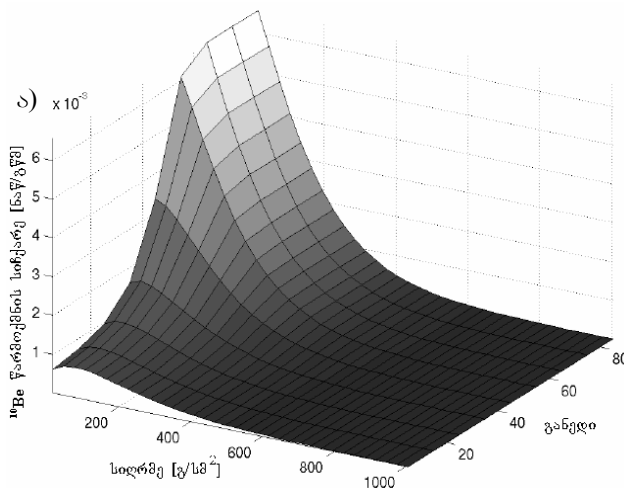
ნახ 29 ა) კოსმოგენური ^{10}Be ის წარმოქმნის სიჩქარის დამოკიდებულება გეოგრაფიულ განედსა და ატმოსფეროს “სიღრმეზე” ბ) რადიონახშირბადის წარმოქმნის სიჩქარის დამოკიდებულება განედზე სხვადასხვა მოდულაციის პარამეტრისას [154,158]
