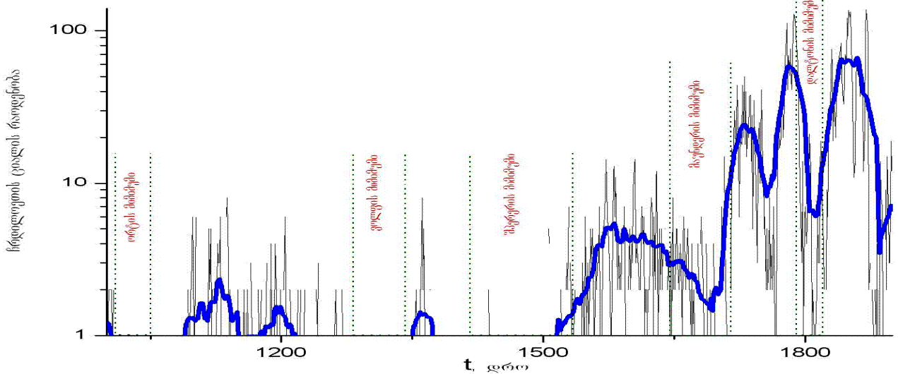
ნახ24. ჩრდილოეთის ციალის რაოდენობა ისტორიულ ცნობებზე დაყრდნობით. მუქი ხაზით ნაჩვენებია 25 წერტილით გასაშუალოებული მრუდი.
