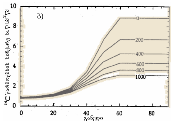
ნახ 29 ა) კოსმოგენური ^{10}Be ის წარმოქმნის სიჩქარის დამოკიდებულება გეოგრაფიულ განედსა და ატმოსფეროს “სიღრმეზე” ბ) რადიონახშირბადის წარმოქმნის სიჩქარის დამოკიდებულება განედზე სხვადასხვა მოდულაციის პარამეტრისას [154,158]
