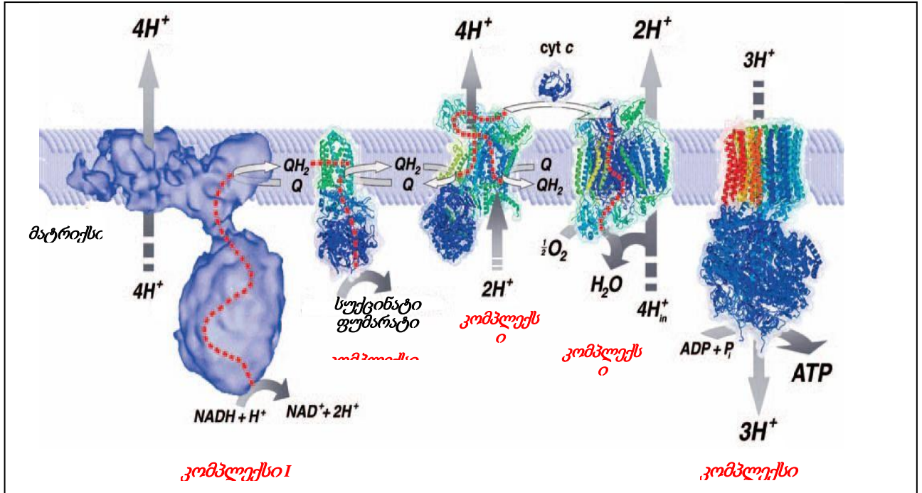
სურ. 1.2.2. მიტოქონდრიული სუნთქვითი ჯაჭვის კომპლექსები და ელექტრონების გადატანის მიმართულება (Nijtmans and Smeitink, 2007)
