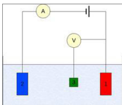
სურათი 2.8. სამელექტროდიანი ვოლტამპერომეტრული უჯრედის სქემატური აგებულება (ა) და ტიპური ვოლტამპერომეტრული სიგნალი (ბ). 1 - მუშა ელექტროდი; 2 - დამხმარე ელექტროდი; 3 - შედარების ელექტროდი; 4 - კვების წყარო.
