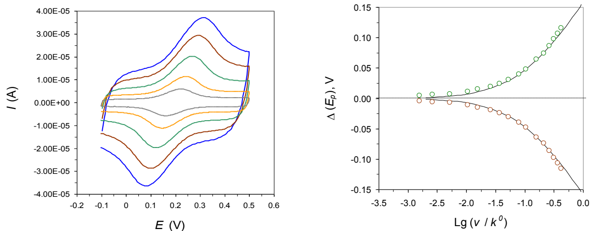
სურათი 2.9. (a) Au/SAM/Az სისტემაში ელექტრონის გადატანის შესაბამისი ვოლტამოგრამები. 70% [ch][dhp], pH 4.6, T = 20^\circ C , P = 0.1 MPa , პოტენციალის სკანირების სიჩქარეები: 10, 20, 40, 60 და 80 V s^{-1} . (b) მიღებული პიკების დაშორებების როგორც სკანირების სიჩქარის ფუნქციის ფიტინგი მარკუსის მოდელის მიხედვით. მიღებული პარამეტრები k^0 = 190 s^{-1} , \lambda = 0.3 eV .
