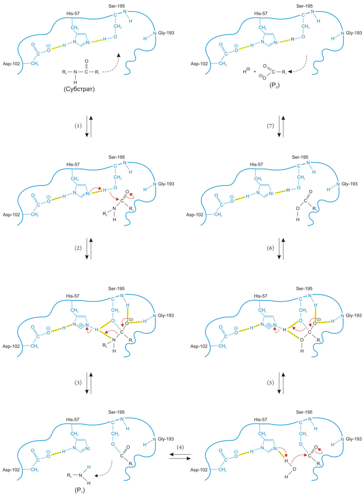
სურათი 1.7. α-ქიმოტრიფსინისათვის დამახასიათებელი პეპტიდის ჰიდროლიზის რეაქციის ელემენტარული სტადიები.
