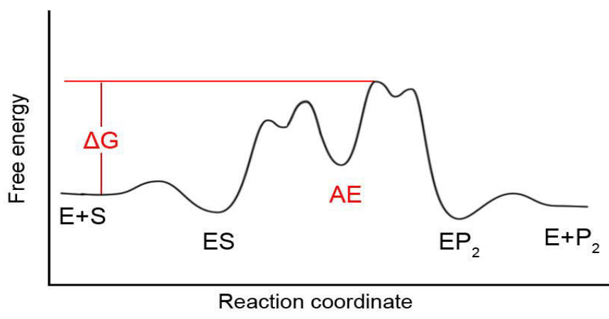
სურათი 1.6. ATEE-ს ჰიდროლიზის პროცესის თავისუფალი ენერგია.
