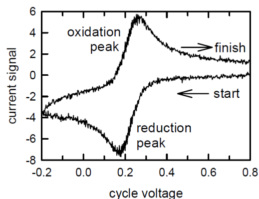
სურათი 2.8. სამელექტროდიანი ვოლტამპერომეტრული უჯრედის სქემატური აგებულება (ა) და ტიპური ვოლტამპერომეტრული სიგნალი (ბ). 1 - მუშა ელექტროდი; 2 - დამხმარე ელექტროდი; 3 - შედარების ელექტროდი; 4 - კვების წყარო.
