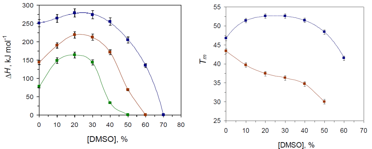
სურათი 3.5 თერმული დენატურაციის ენტალპიის და ტემპერატურის დამოკიდებულება ხსნარში DMSO-ს კონცენტრაციაზე pH-ის ორი სხვადასხვა მნიშვნელობის დროს (შესაბამისად, pH 2.6 და 8.1); pH 2.6-ის შემთხვევაში გადასვლის ენტალპიები ნაჩვენებია პირველი და გამეორებული სკანირების შემთხვევებში.
