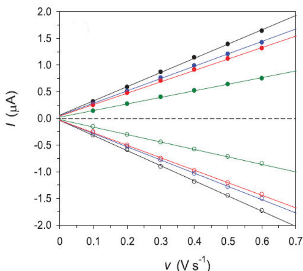
სურათი 3.12 Au/Cys SAM/Cu სისტემის მიერ ელექტრონის მიმოცვლის შესაბამისი პიკის დენის დამოკიდებულება სკანირების სიჩქარეზე სხვადასხვა pH-ის პირობებში. 0.1 M PBS, pH 6.5, 6.9, 7.3 და 7.7, T = 20 °C.
