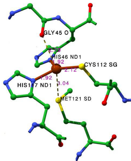
სურათი 1.8. აზურინის აქტიური ცენტრი. წითლად არის ნაჩვენები სპილენძის იონი და მისი ლიგანდები. იისფრად მოცემულია მანძილები სპილენძის იონისა და ლიგანდებამდე ანგსტრემებში.
