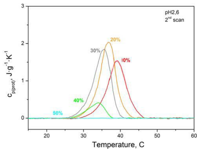
სურათი 3.3. გამეორებული სკანირების შედეგად მიღებული \alpha -ქიმოტრიპსინის თერმული ლღობის კალორიმეტრული მრუდები ხსნარში DMSO-ს სხვადასვა კონცენტრაციის პირობებში (ფოსფატის ბუფერი, pH 2.6, 0.05 NaCl).
