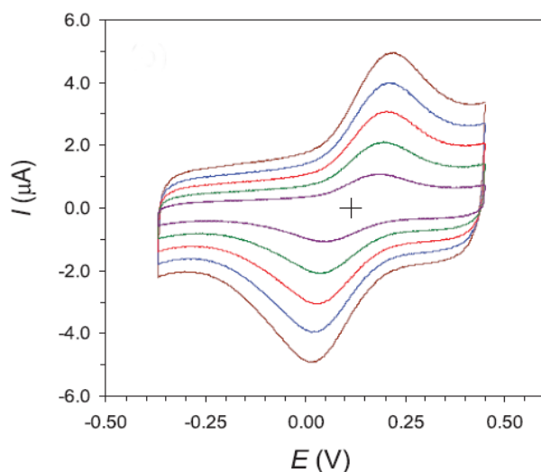
სურათი 3.13 Au/Cys SAM/Cu სისტემის მიერ ელექტრონის გადატანის პროცესის ტიპური ვოლტამოგრამა. სკანირების სიჩქარეები 0.1 – 1 V·s -1 (0.1 M PBS, pH 5.7).
